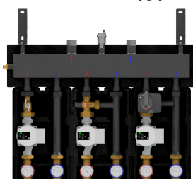
Zestaw DX 132 - zestaw 3 obiegów grzewczych - jeden bez zaworu mieszającego, jeden z termostatycznym zaworem mieszającym oraz jeden z mieszającym zaworem obrotowym i siłownikiem elektrycznym
