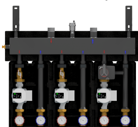
Zestaw DX 113 - zestaw 3 obiegów grzewczych - dwa bez zaworów mieszających oraz jeden z termostatycznym zaworem mieszającym
