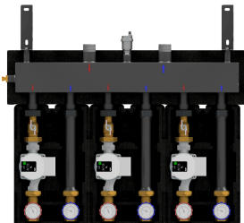
Zestaw DX 112 - zestaw 3 obiegów grzewczych - dwa bez zaworów mieszających oraz jeden z mieszającym zaworem obrotowym i siłownikiem elektrycznym
