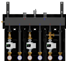
Zestaw DX 122 - zestaw 3 obiegów grzewczych - jeden bez zaworu mieszającego oraz dwa z mieszającymi zaworami obrotowymi i siłownikami elektrycznymi
